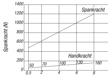
Zwenkspanner K0912....4540
