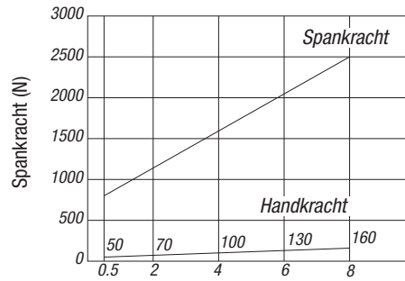
Trekspanner K0910.4050...
